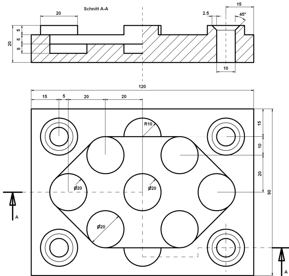
Werkstück: Lochplatte
