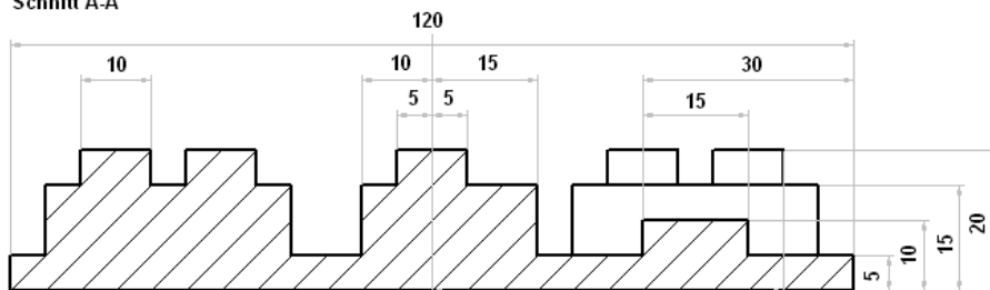
Schnitt A-A
